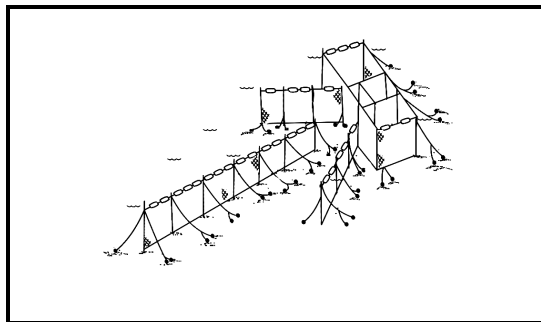
Fig. 32. Set net
