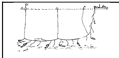
Fig. 37. Set long line
