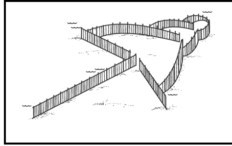
Fig. 34. Corral
